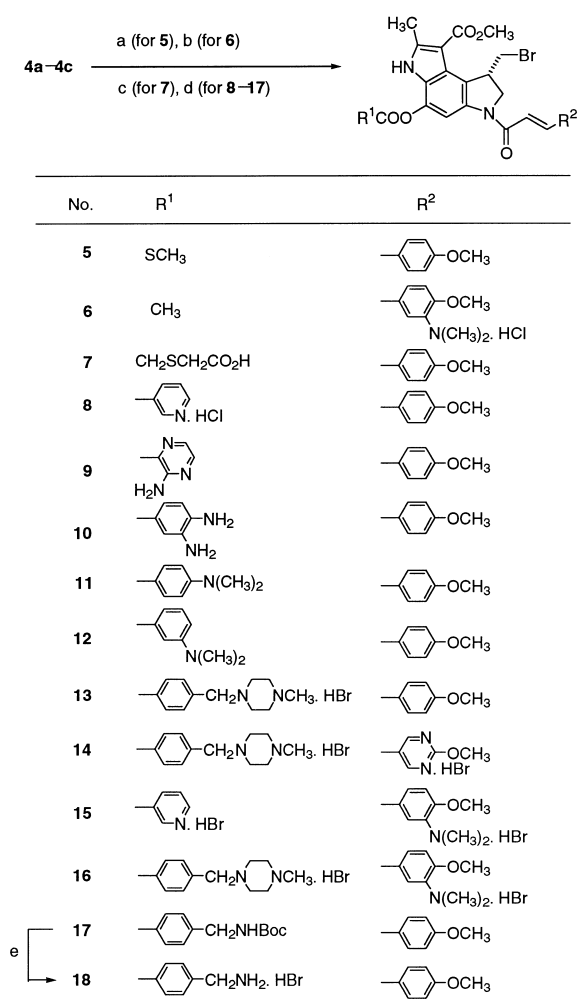
Scheme 2. (a) (1) HBr, CH 3 CN, (2) CH 3 SCl, Et 3 N, CH 2 Cl 2 ; (b) (1) HBr, CH 3 CN, (2) Ac 2 O, 4-dimethylaminopyridine (DMAP), CH 2 Cl 2 , (3) HCl; (c) (1) HBr, CH 3 CN, (2) thiodiglycolic anhydride, DMAP, CH 2 Cl 2 , (d) (1) HBr, CH 3 CN, (2) R 1 CO 2 H, DCC, DMAP, CH 2 Cl 2 , (3) HCl for 8 or HBr for 13–16; (e) (1) HBr, ClCH 2 CH 2 Cl, 60 °C, (2) HBr.
